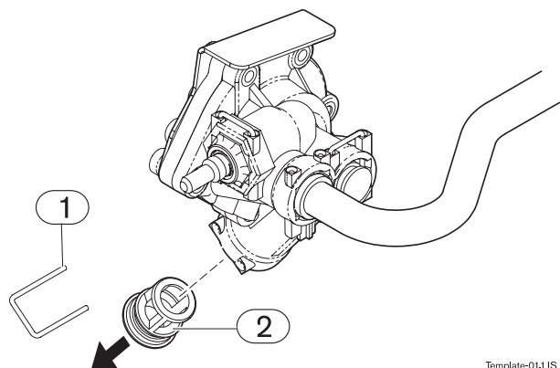
Рис 14 Опорожнение прибора
